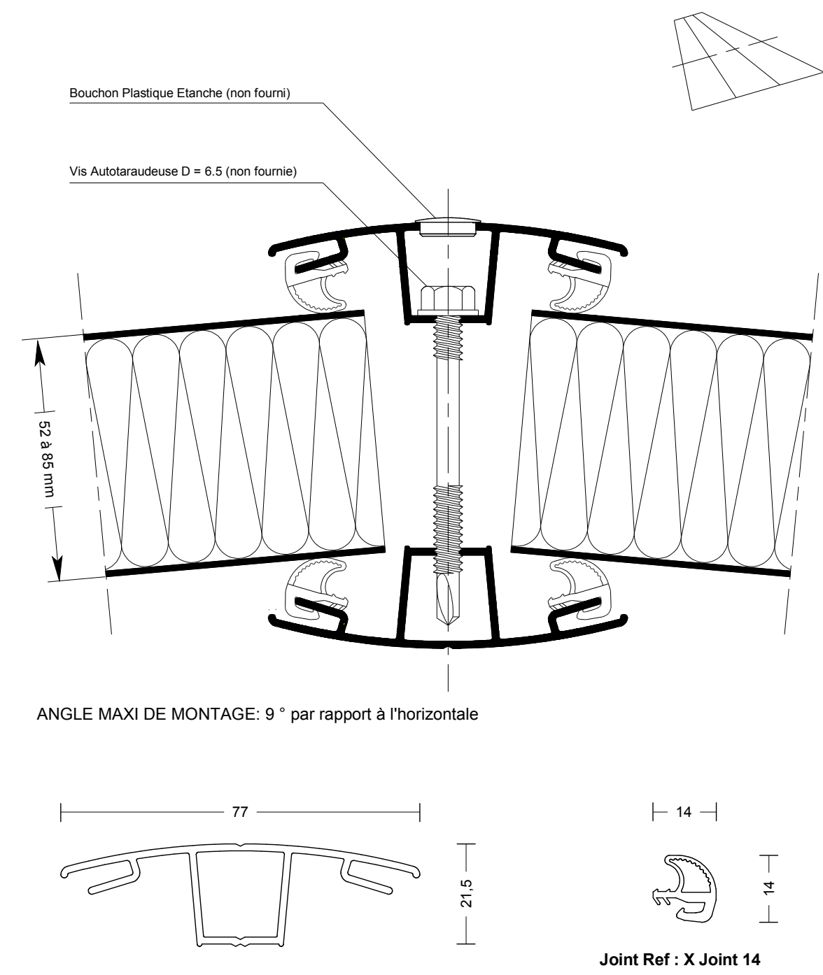
Profilé ALUMINIUM Ref : E 4549
