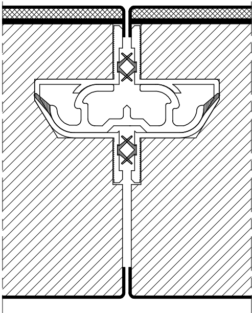
EPAISSEUR 85 mm AST CONFORT
