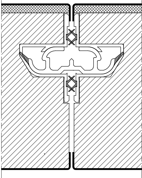
EPAISSEUR 85 mm AST PREMIUM
