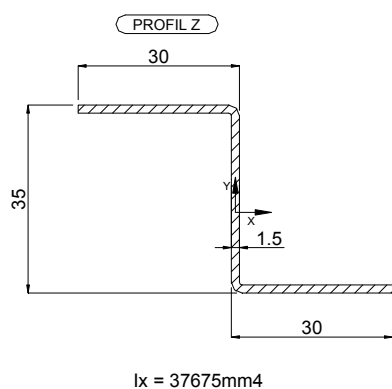
Figure 28 – Profilés en acier galvanisé 15/10 mini
