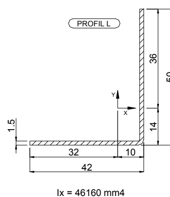
Figure 28 – Profilés en acier galvanisé 15/10 mini
