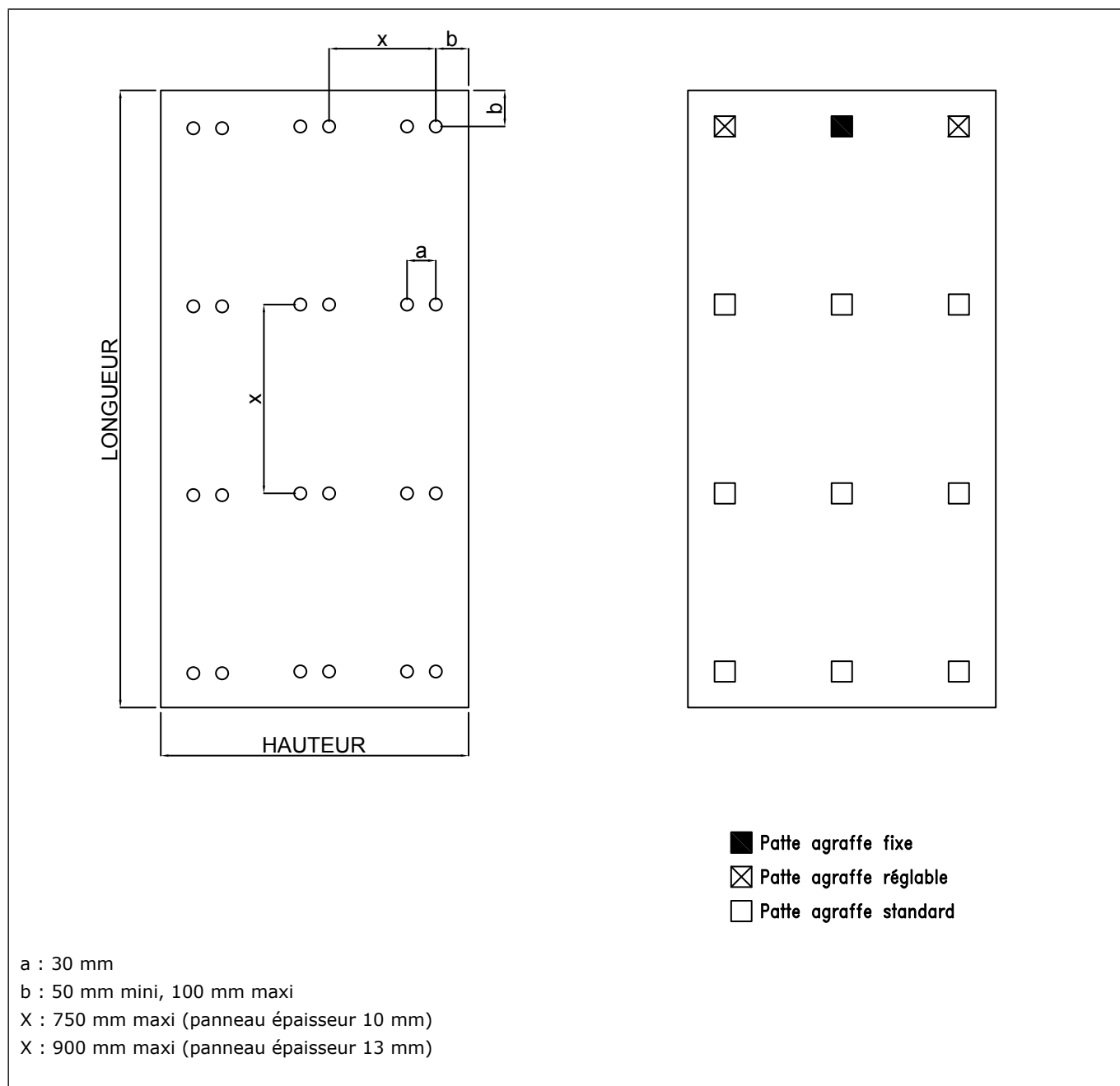
Figure 24bis– Implantation des agrafes pour pose verticale
